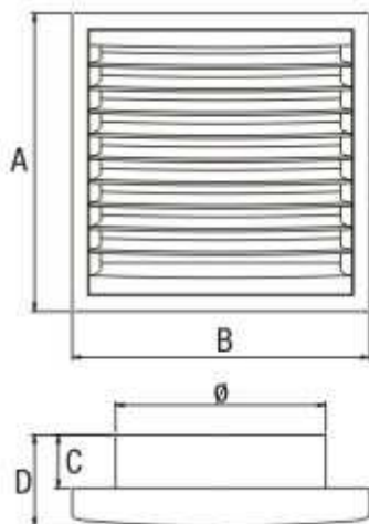
Typ Pevná mriežka B-15
